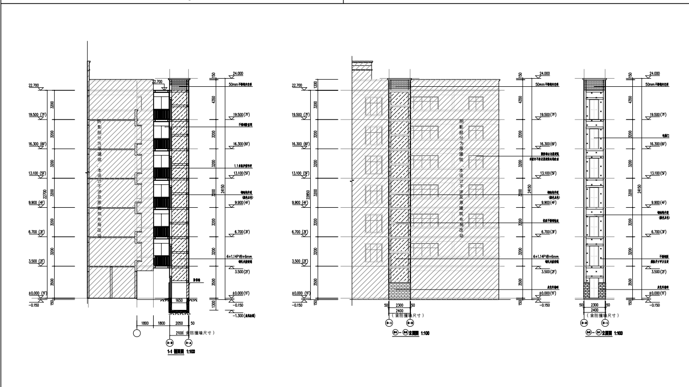
拟建电梯电梯（连廊）立面图、剖面图
