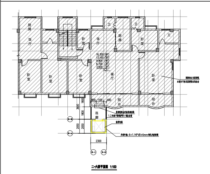
标准层平面图
