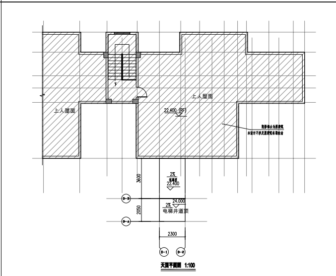
天面层平面图
