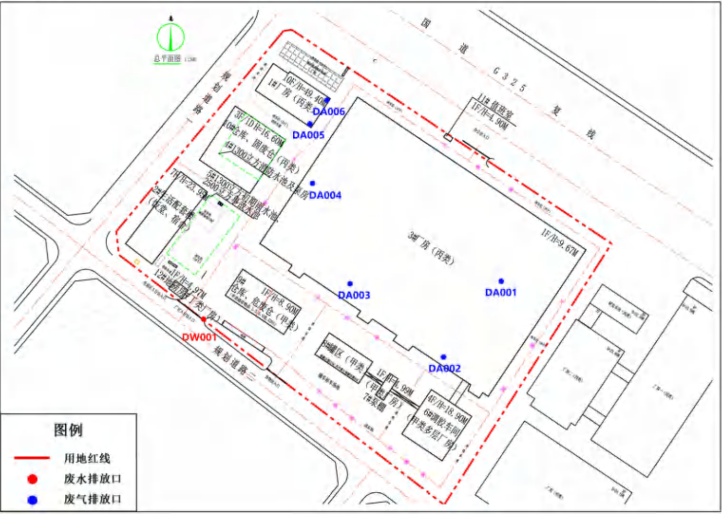
附图 4 本项目总平面布置图
