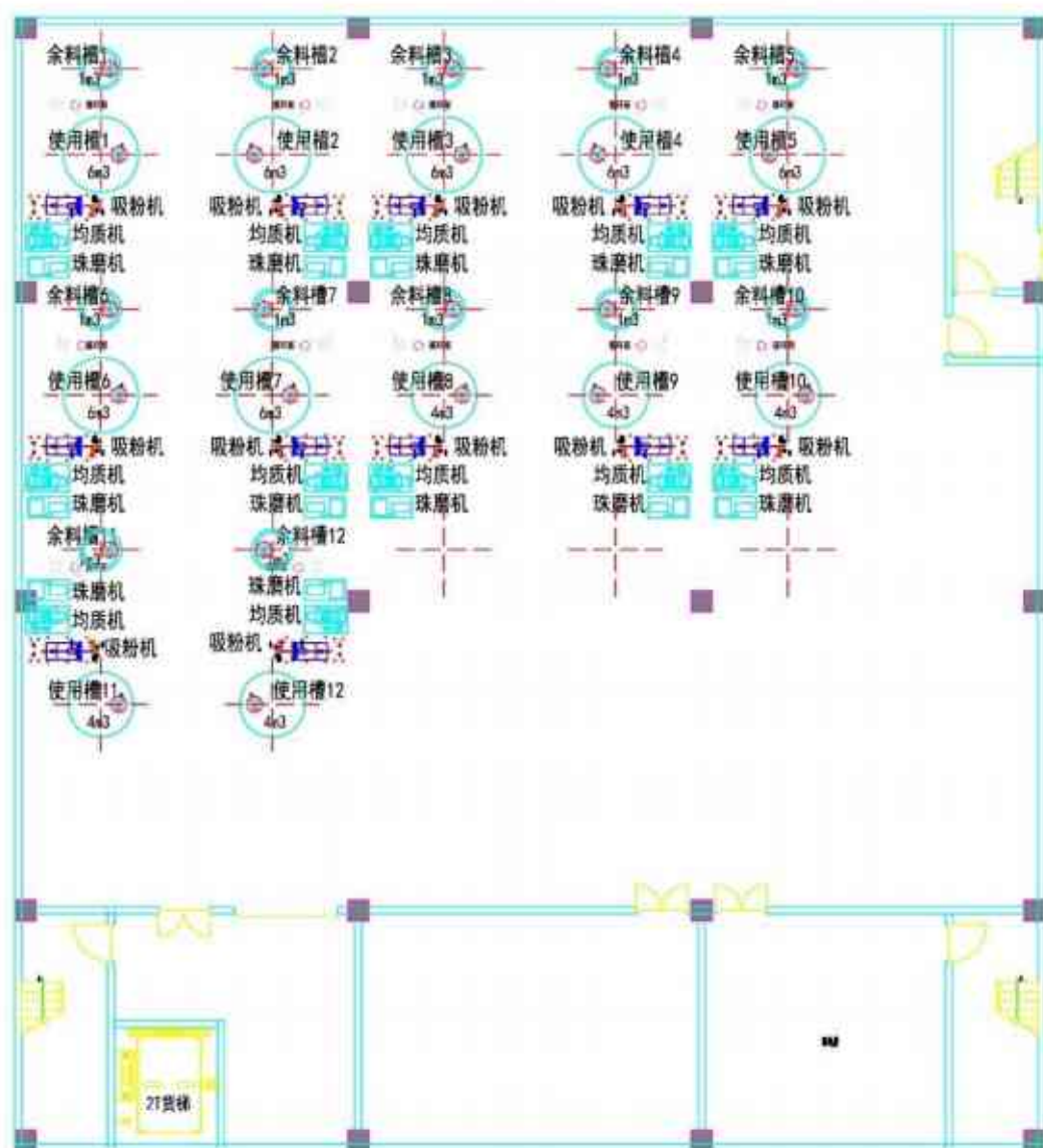
附图 5.2 6#调胶车间 2F 设备布局图
