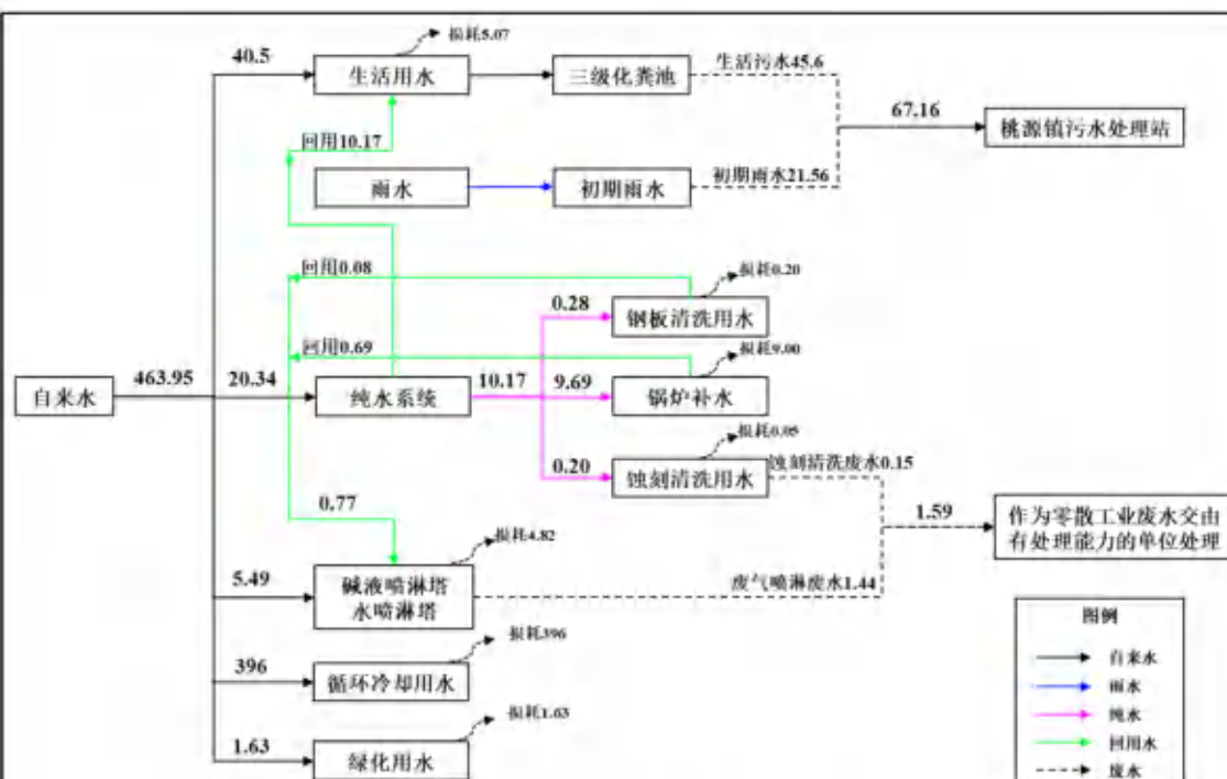
图 2.5-1 本项目水平衡图 (单位: \text{m}^3/\text{d} )
