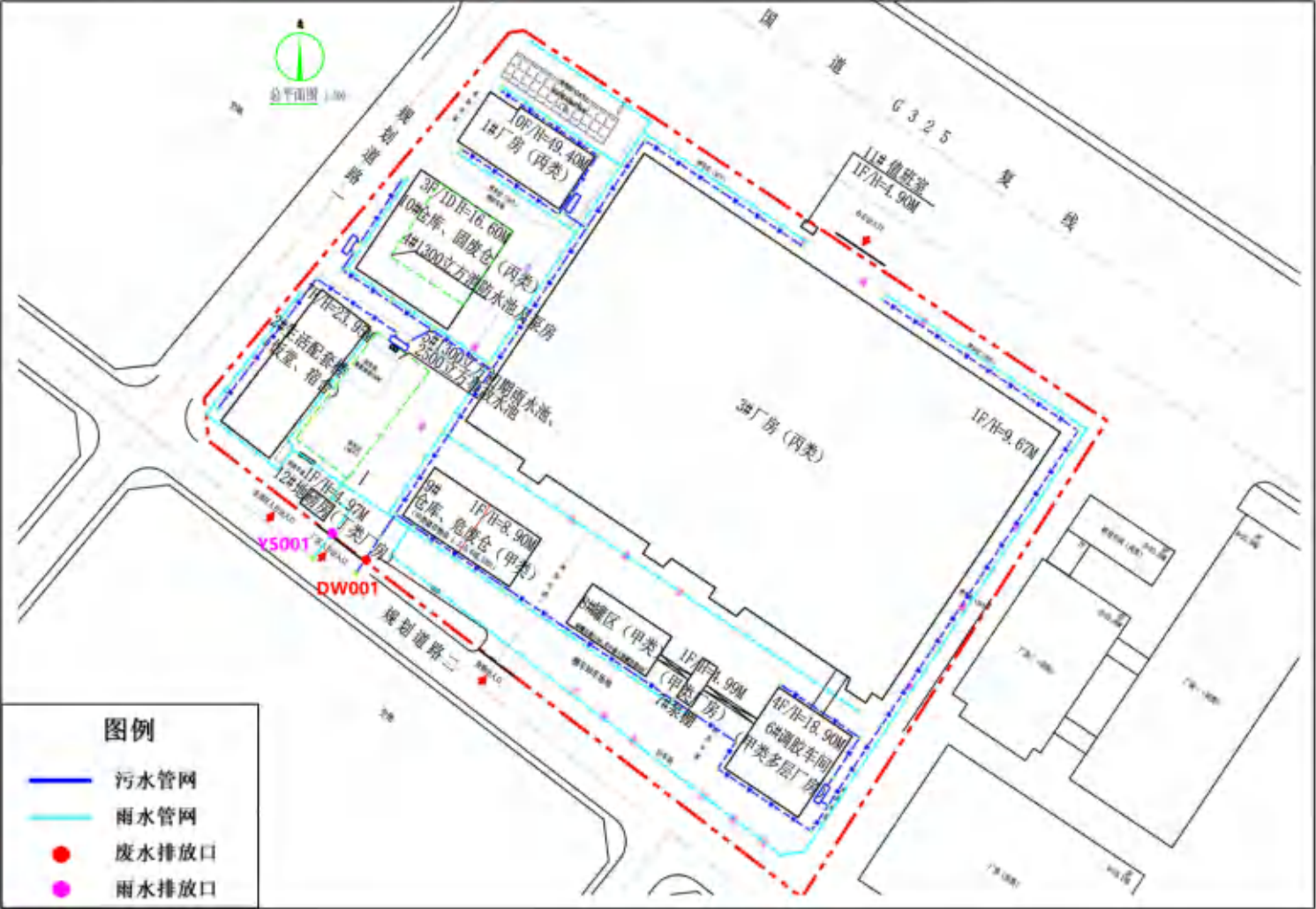
附图 6 本项目全厂雨污管网分布示意图
