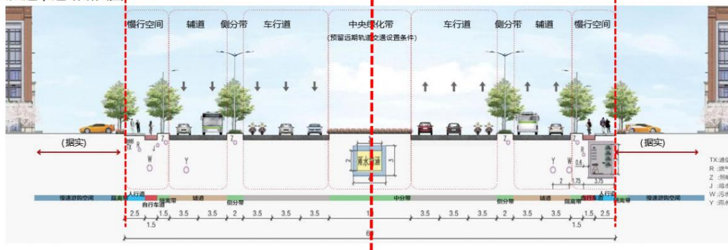
2. 鹤山大道（人民东路-龙口大道）道路断面图
