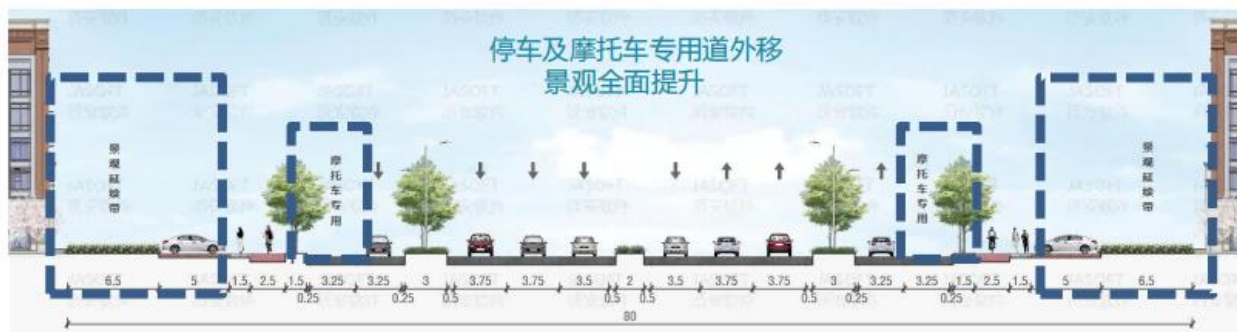
远期改善方案
