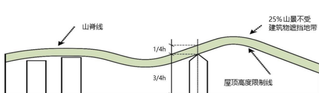
山边建筑高度控制示意图
