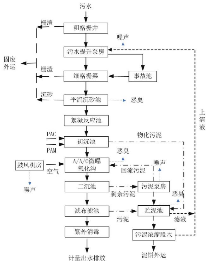
图 10. 鹤山产业转移园址山片区污水处理厂处理工艺流程图
