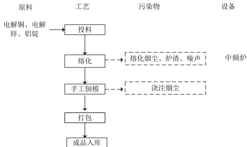
图 4. 铝黄铜锭生产工艺流程图
