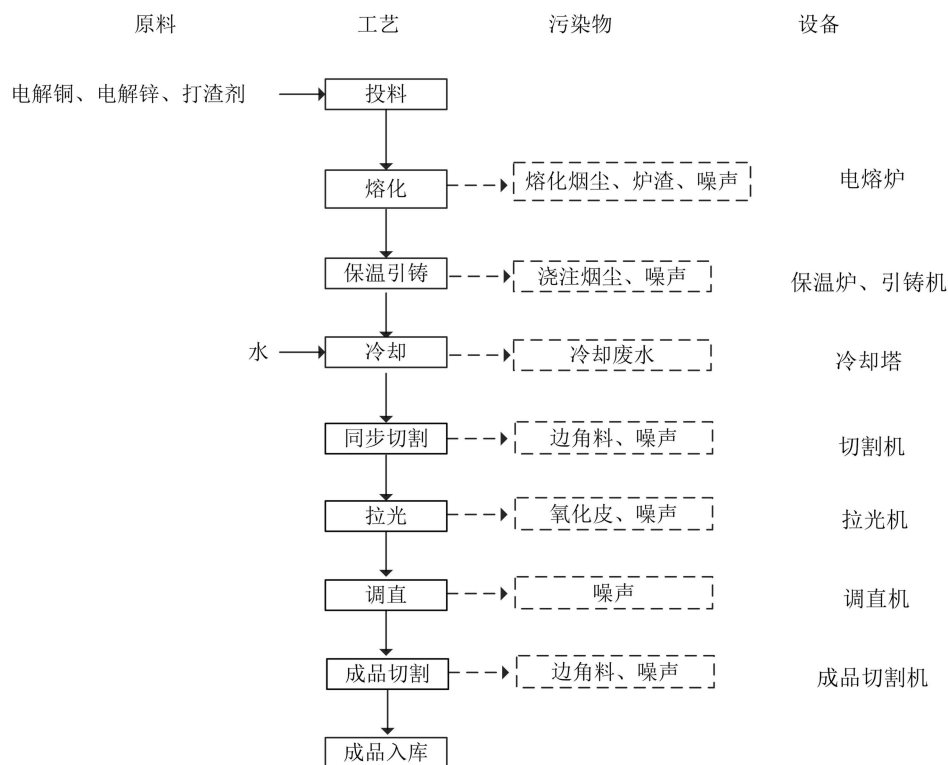
图 3. 普通黄铜棒生产工艺流程图
