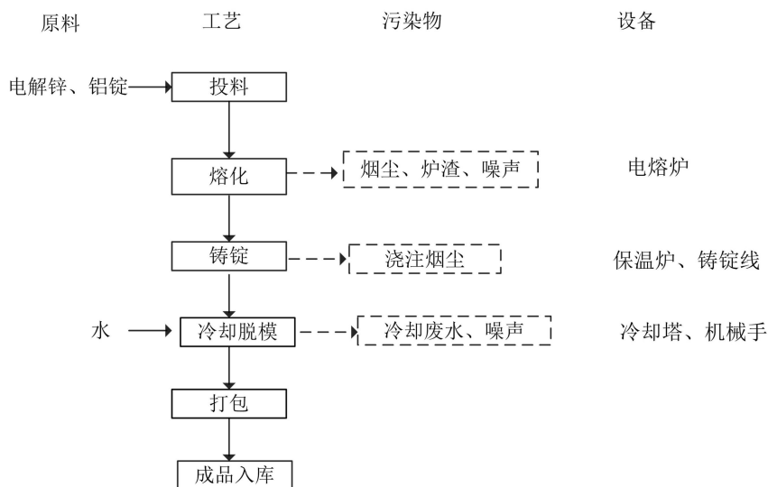
图 5. 锌合金锭生产工艺流程图
