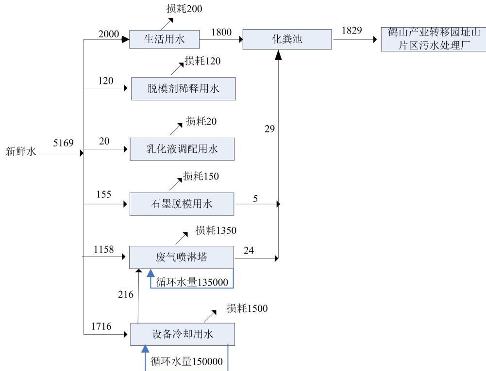
图 2. 项目水平衡图 (t/a)
