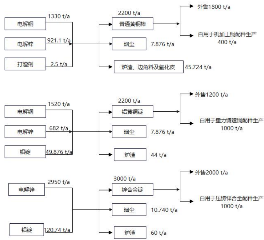
图 1. 项目合金生产工序物料平衡图
