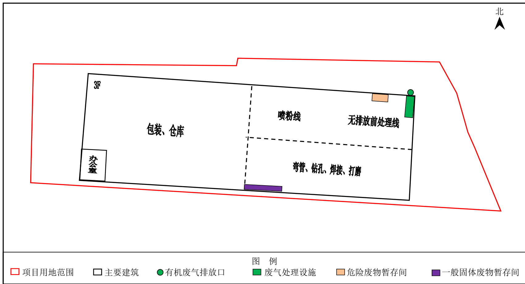
附图 4 项目厂房 3 楼平面布置图
