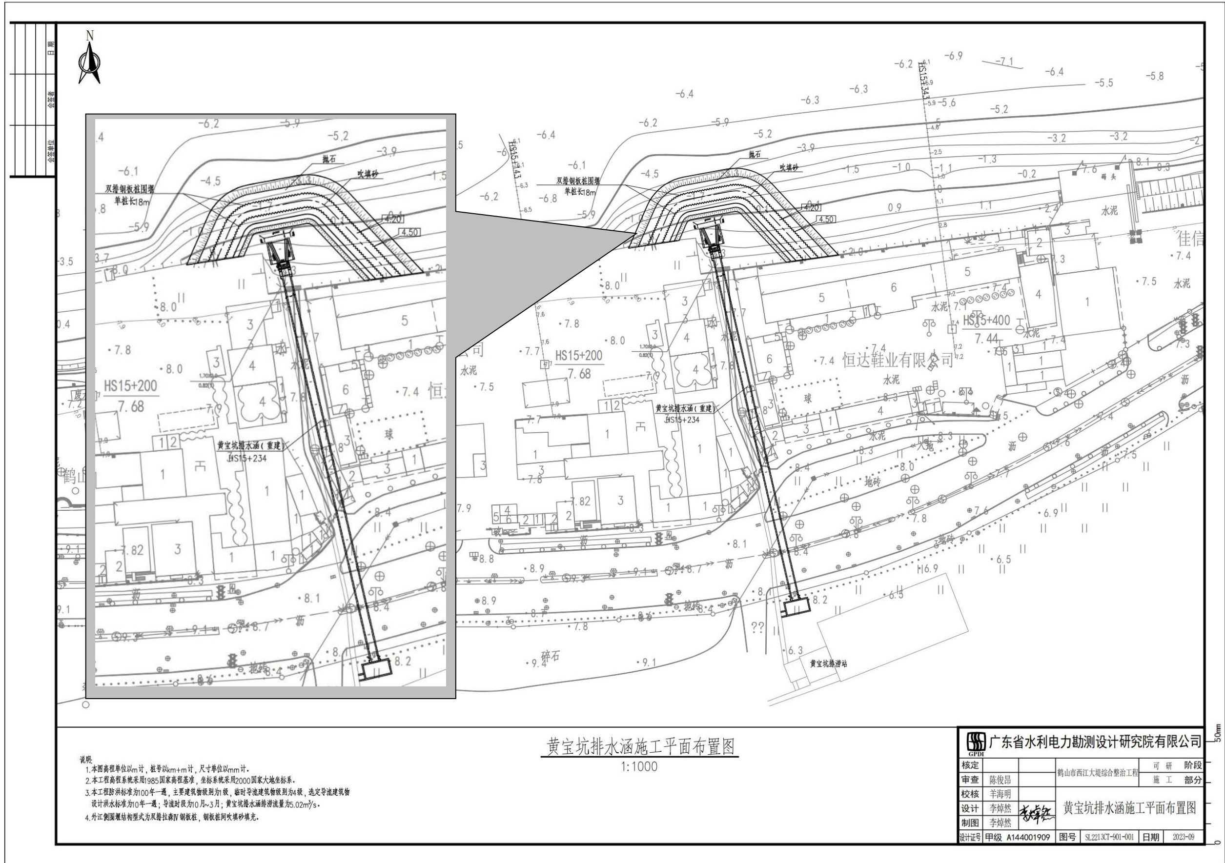
附图 15.1 项目施工平面布置图-黄宝坑排水涵
