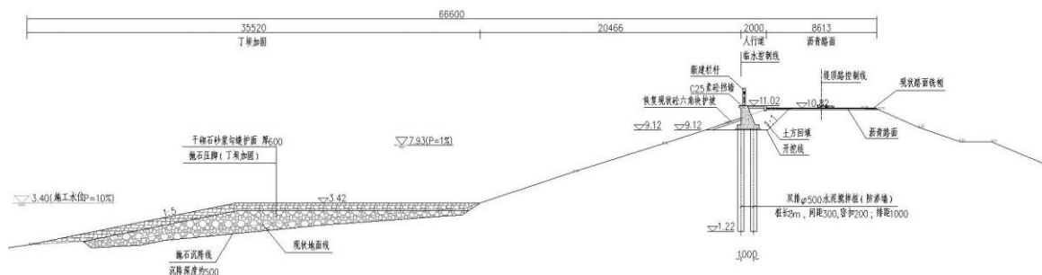
图2-2标准断面图（HS0+346~HS0+743）
