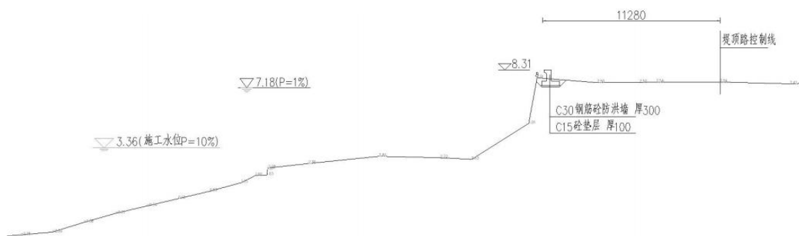
图 2-7 标准断面图（HS12+861~HS13+460）
